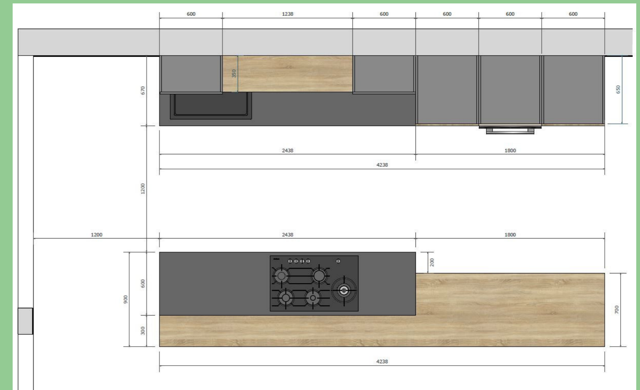
Plan détail cuisine
