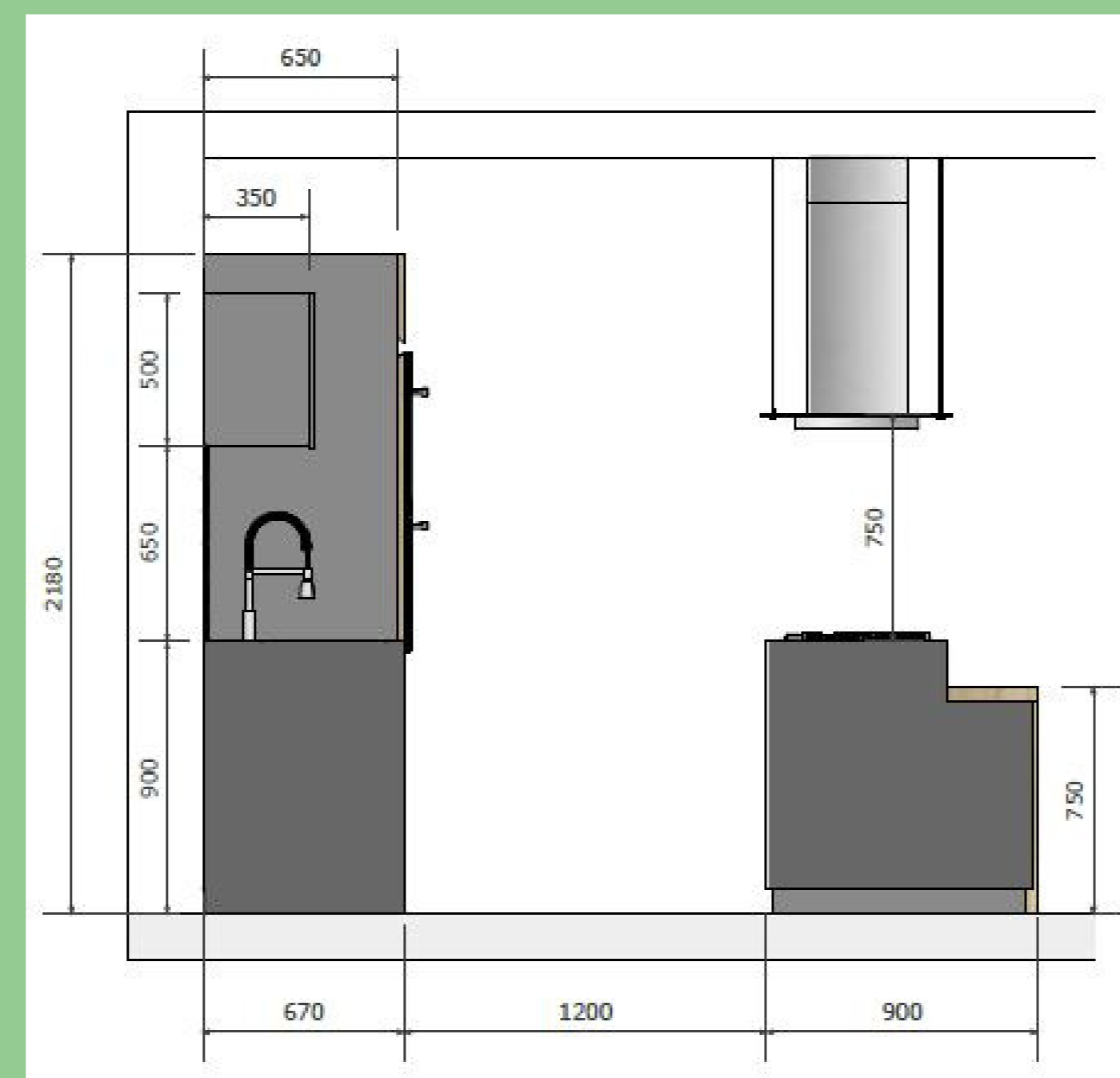
Plan détail cuisine
