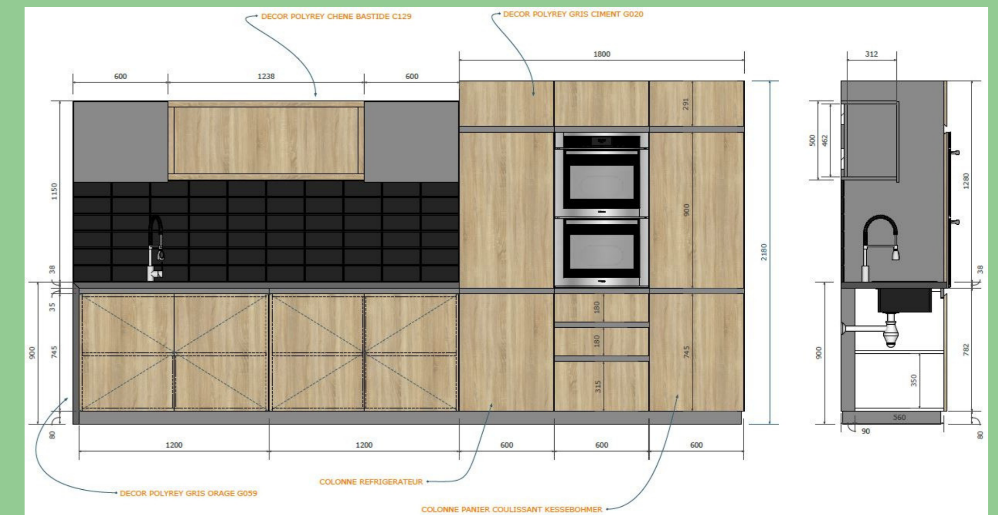
Plan vue cuisine
