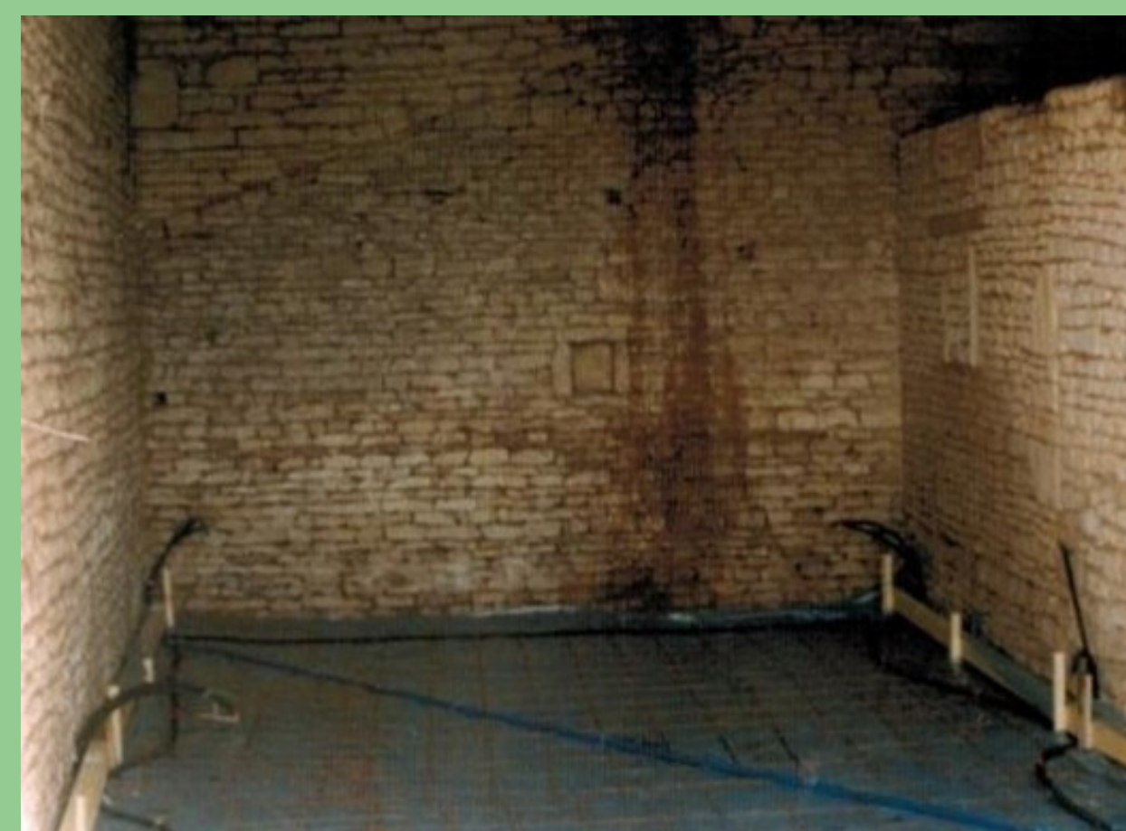
Aménagement d'une grange – plancher chauffant
